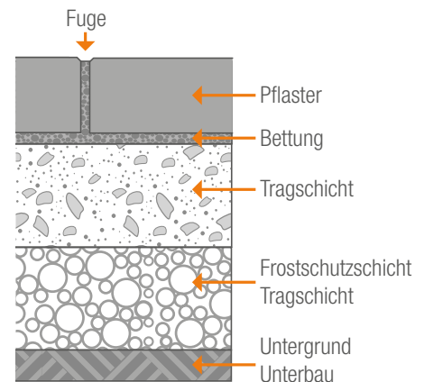
Schematischer Aufbau einer Betonpflasterfläche
