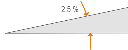
Mindestgefälle des Planums
